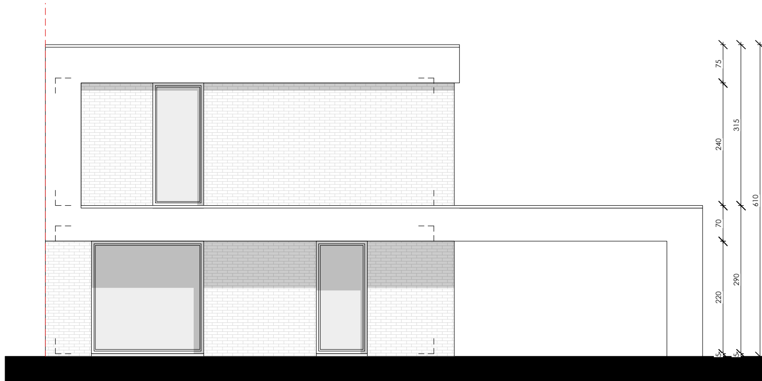
Vorgevel schaal 1/75
